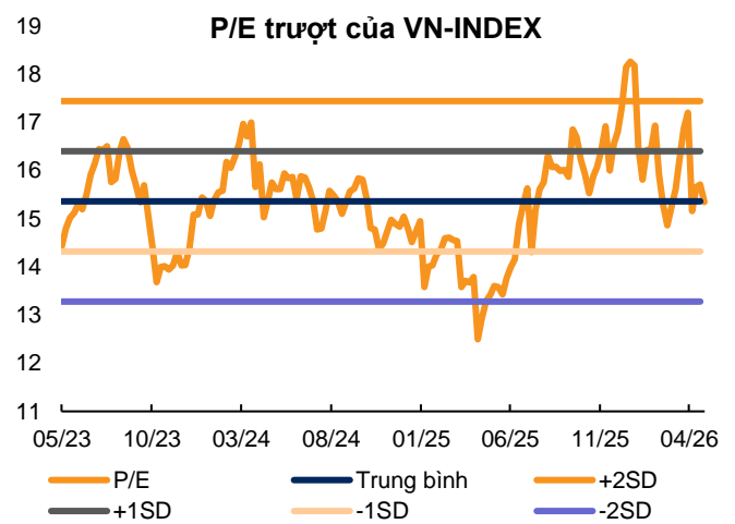
Hình 11: P/E TRƯỢT
